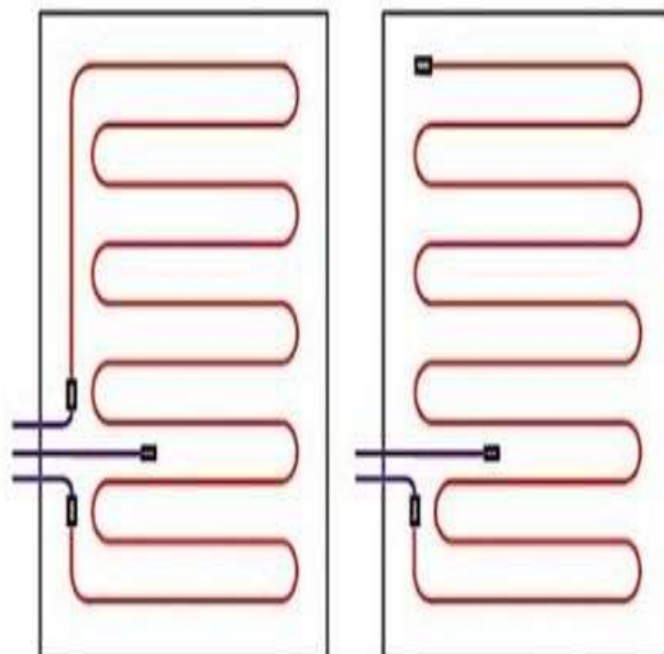
Укладка одножильного кабеля
